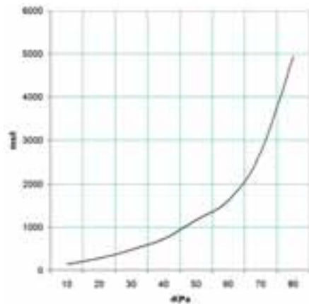
Tiempo de evacuación (ms/l=s/m³) según el grado de vacío (-Kpa)
