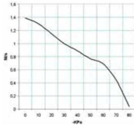
Caudal de aire (NI/s) según el grado de vacío (-Kpa)
