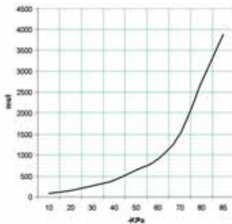
Tiempo de evacuación (ms/l=s/m³) según el grado de vacío (-Kpa)
