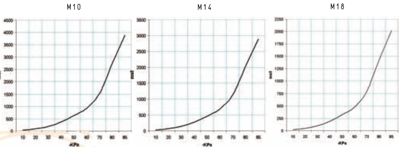
Tiempo de evacuación (ms/l=s/m³) según el grado de vacío (-KPa)
