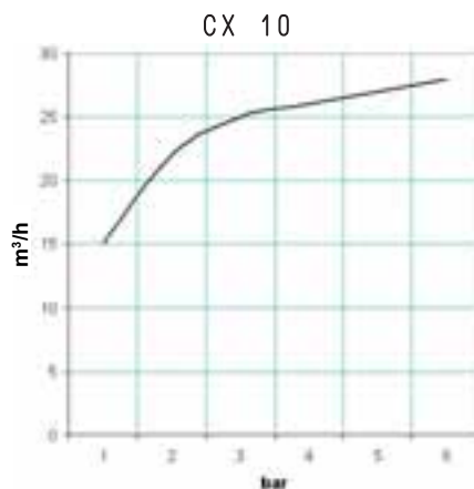
Cantidad de aire soplado (m 3 /h) según la presión de alimentación (bar)
