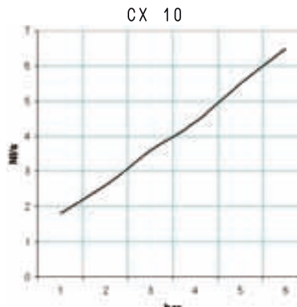
Consumo de aire (NI/s) según la presión de alimentación (bar)
