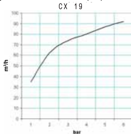
Cantidad de aire soplado (m 3 /h) según la presión de alimentación (bar)
