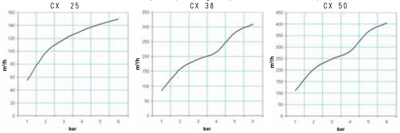
Cantidad de aire soplado (m³/h) según la presión de alimentación (bar)
