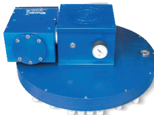
mm Ø400 con soporte de fijación y electroválvula de corte de vacío - SO DO 40 V
