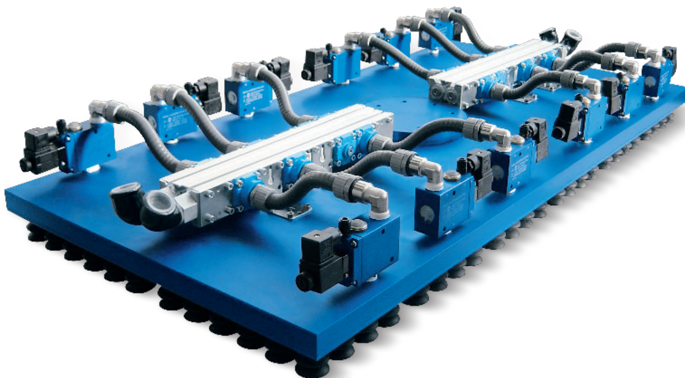
mm 620x1240 con 12 cámaras independientes - SO 62 127 2V
